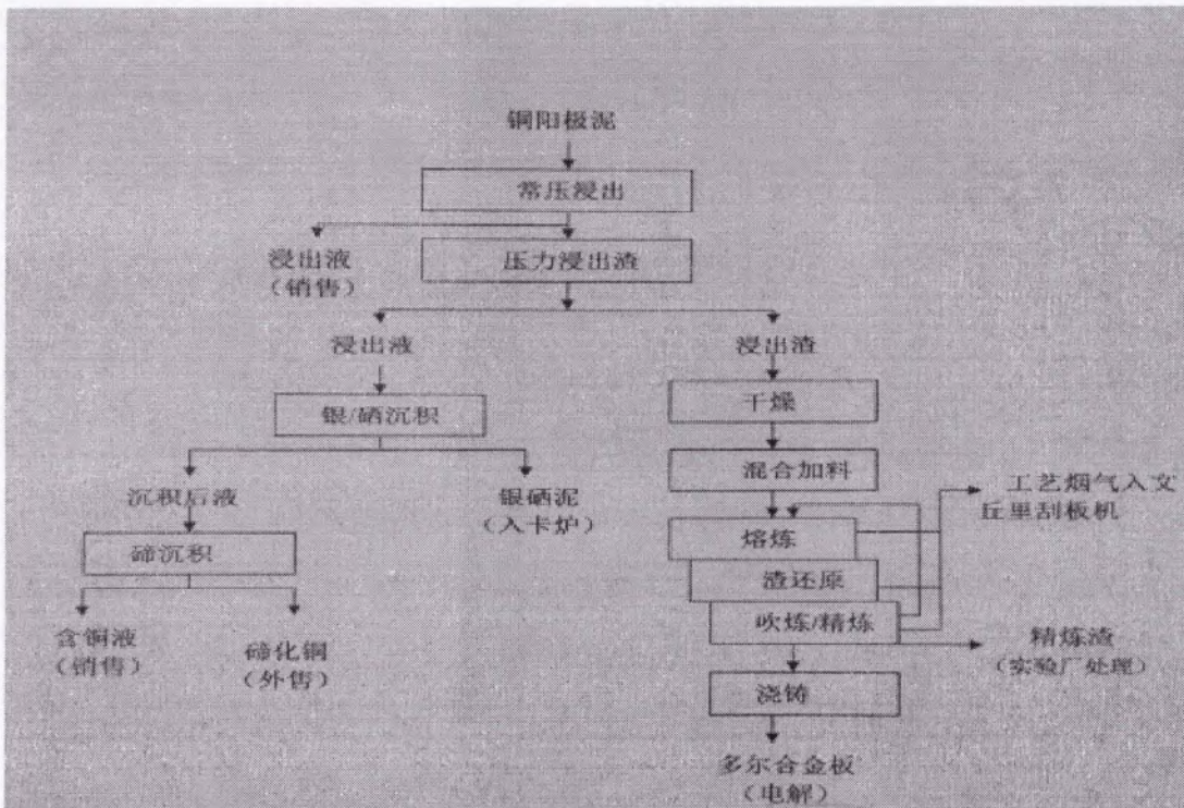
图1 浸出和熔炼工艺
